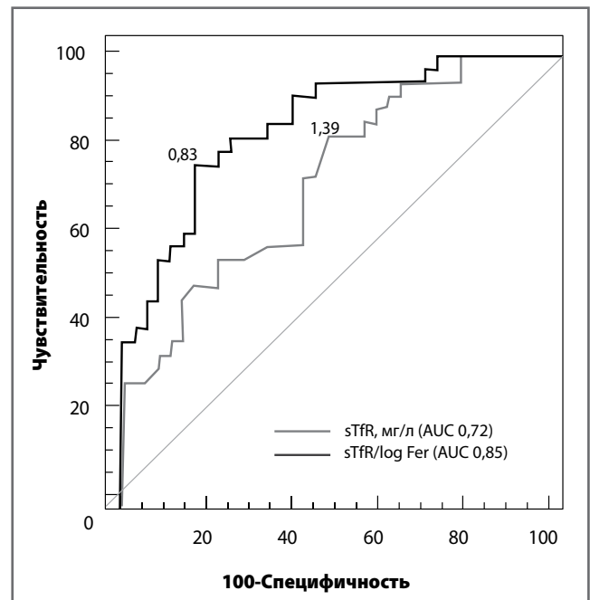
Рис. 1. ROC-кривые для sTfR и sTfR/log Fer.
